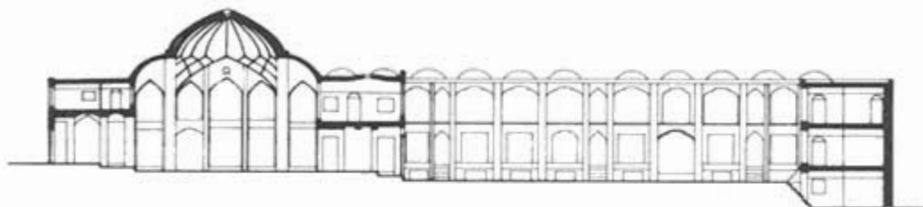
مقطع نمای جنوب A-A
